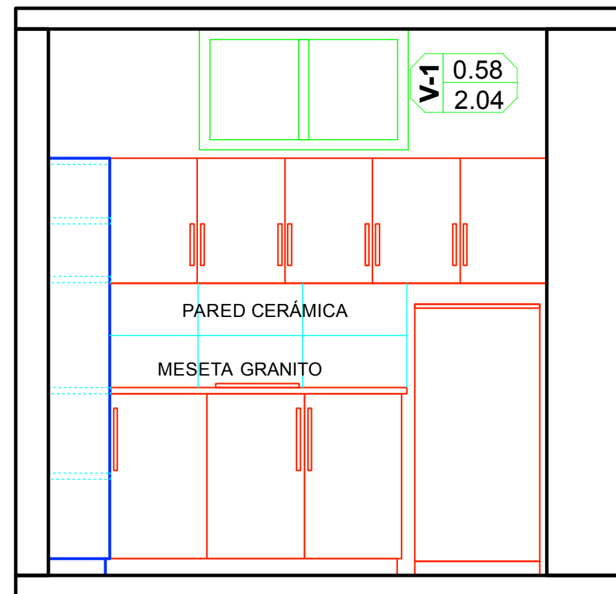
ONESVIE, REGIONAL NORTE ELEVACION 2 / DC
