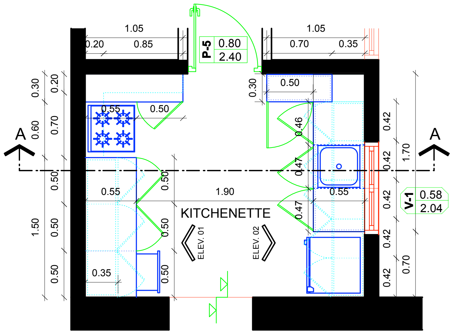
ONESVIE, REGIONAL NORTE DETALLE COCINA DC
