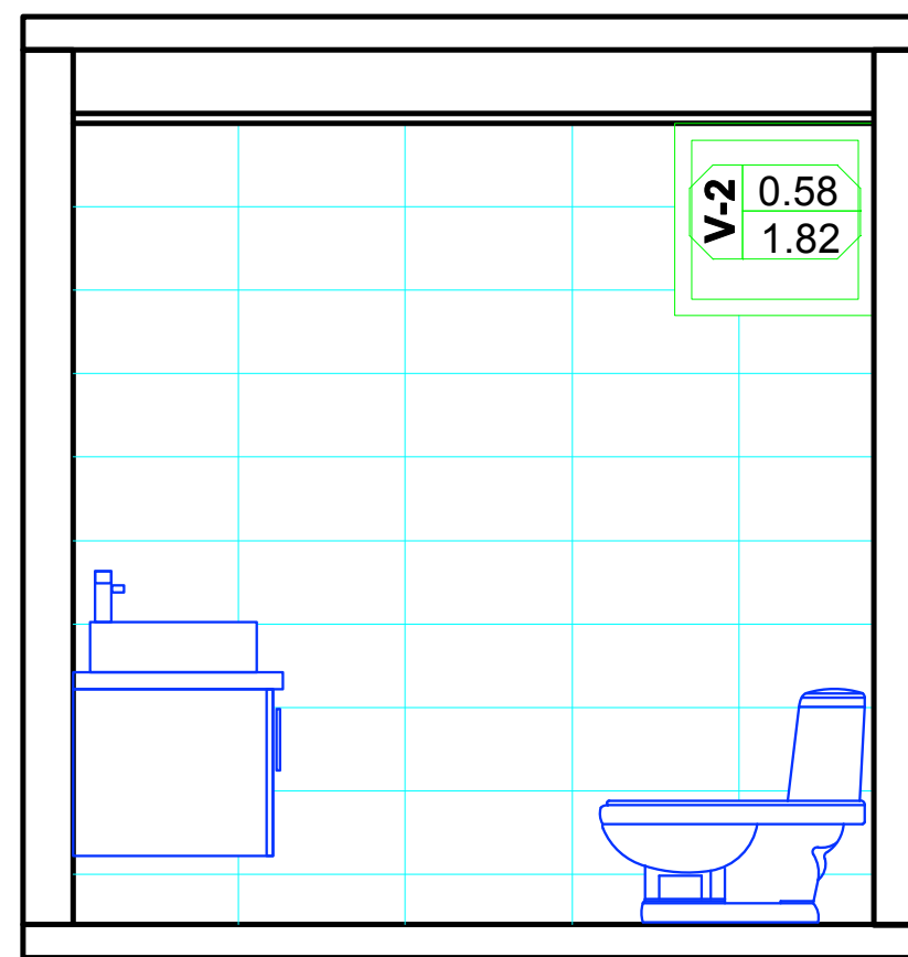
ONESVIE, REGIONAL NORTE ELEVACION 2 / DB
