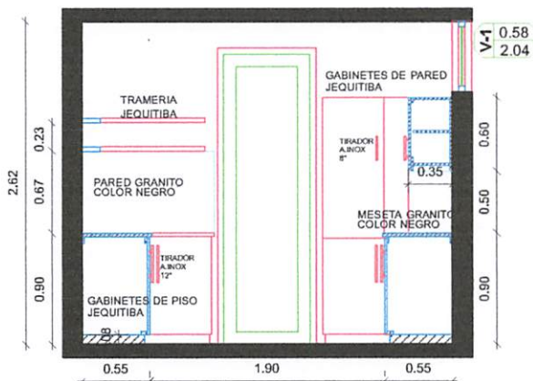
ONESVIE, REGIONAL NORTE SECCION A-A / DC
