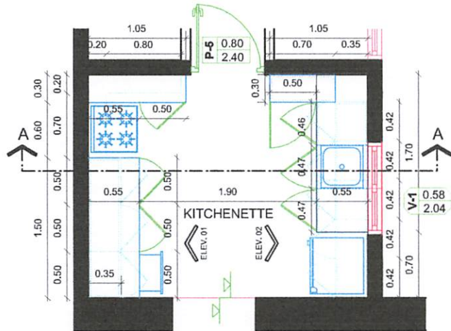
ONESVIE, REGIONAL NORTE DETALLE COCINA DC
